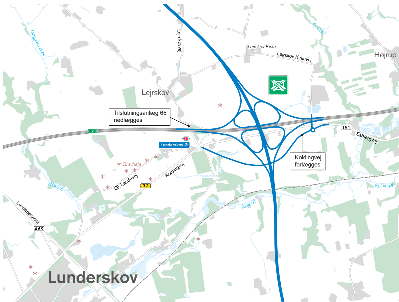
Figur 3.11 Motorvejen ved Lejrskov
