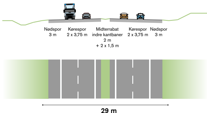
Figur 3.4 Tværsnit for Ny Midtjysk Motorvej ved Give (rute30)
