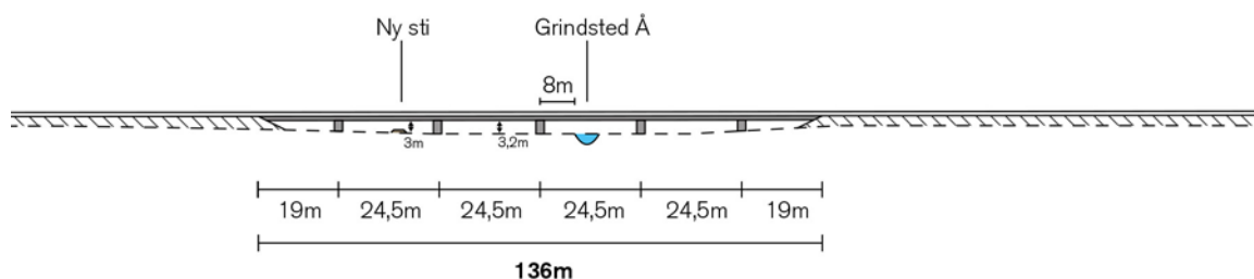
Landskabsbro over Grindsted Å
