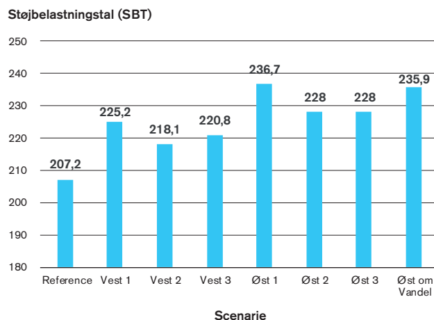
Figur 7.6 Samlet støjbelastningstal (SBT) i undersøgelsesområdet
