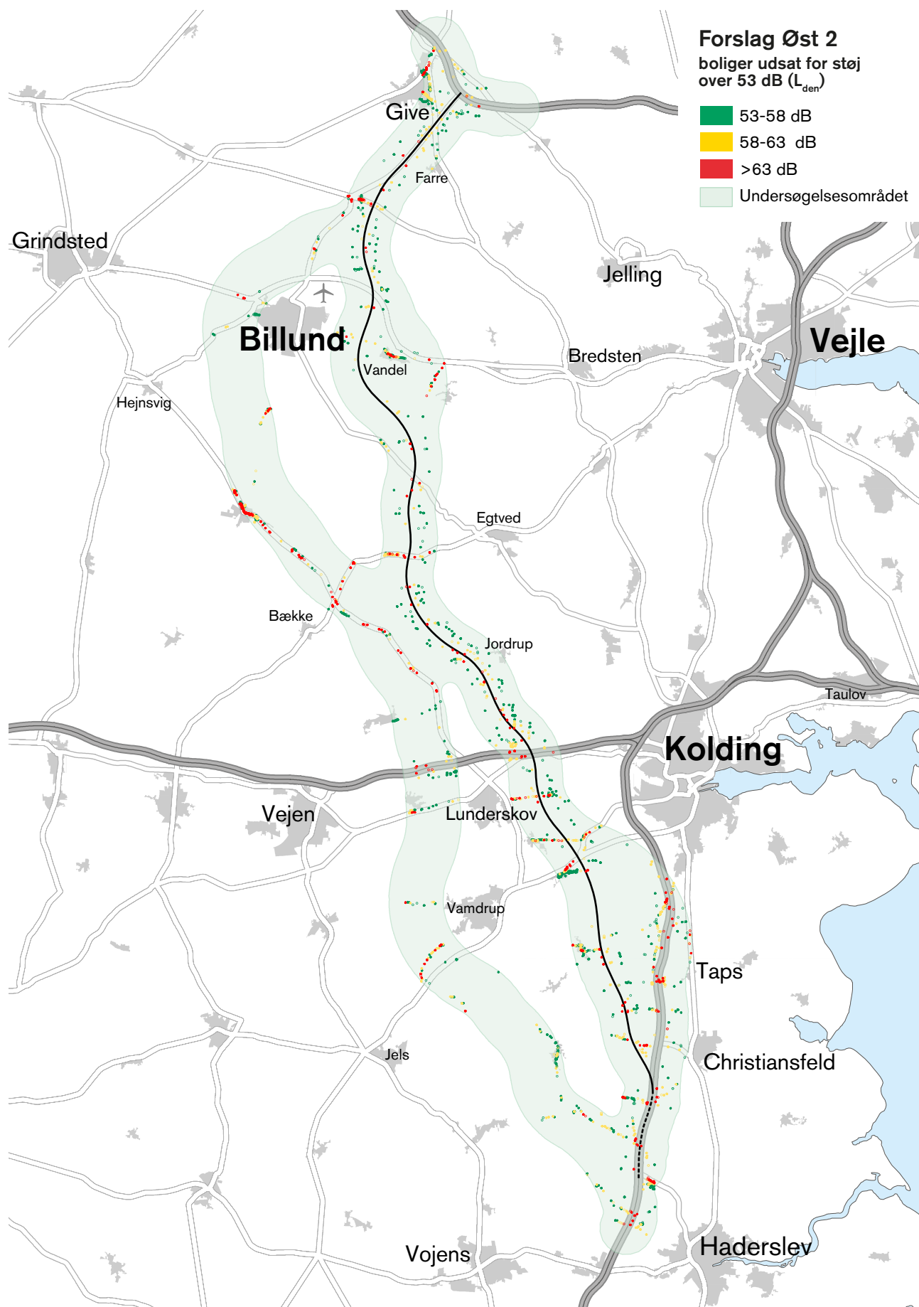
Figur 7.3 Linjeføring ØST 2 – Boliger udsat for støj over 53 dB i undersøgelsesområdet
