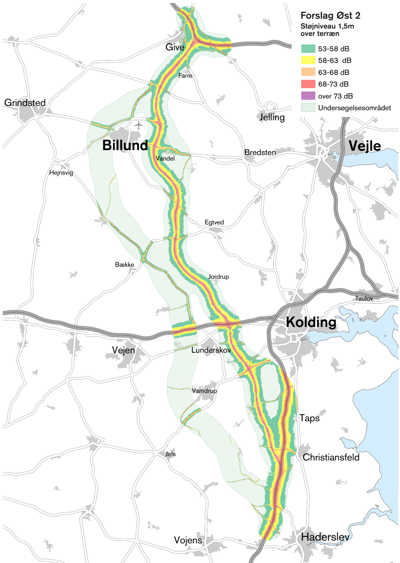
Figur 7.4 Linjeføring ØST 2 – Støjdbredelse indenfor undersøgelsesområdet
