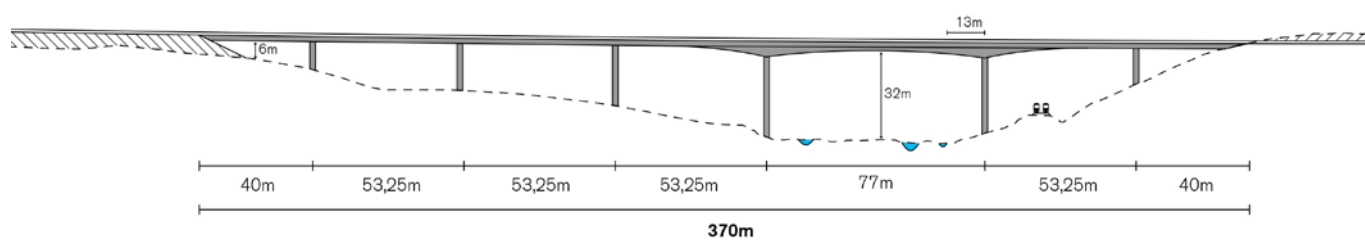
Høj dalbro over Kolding Ådal
