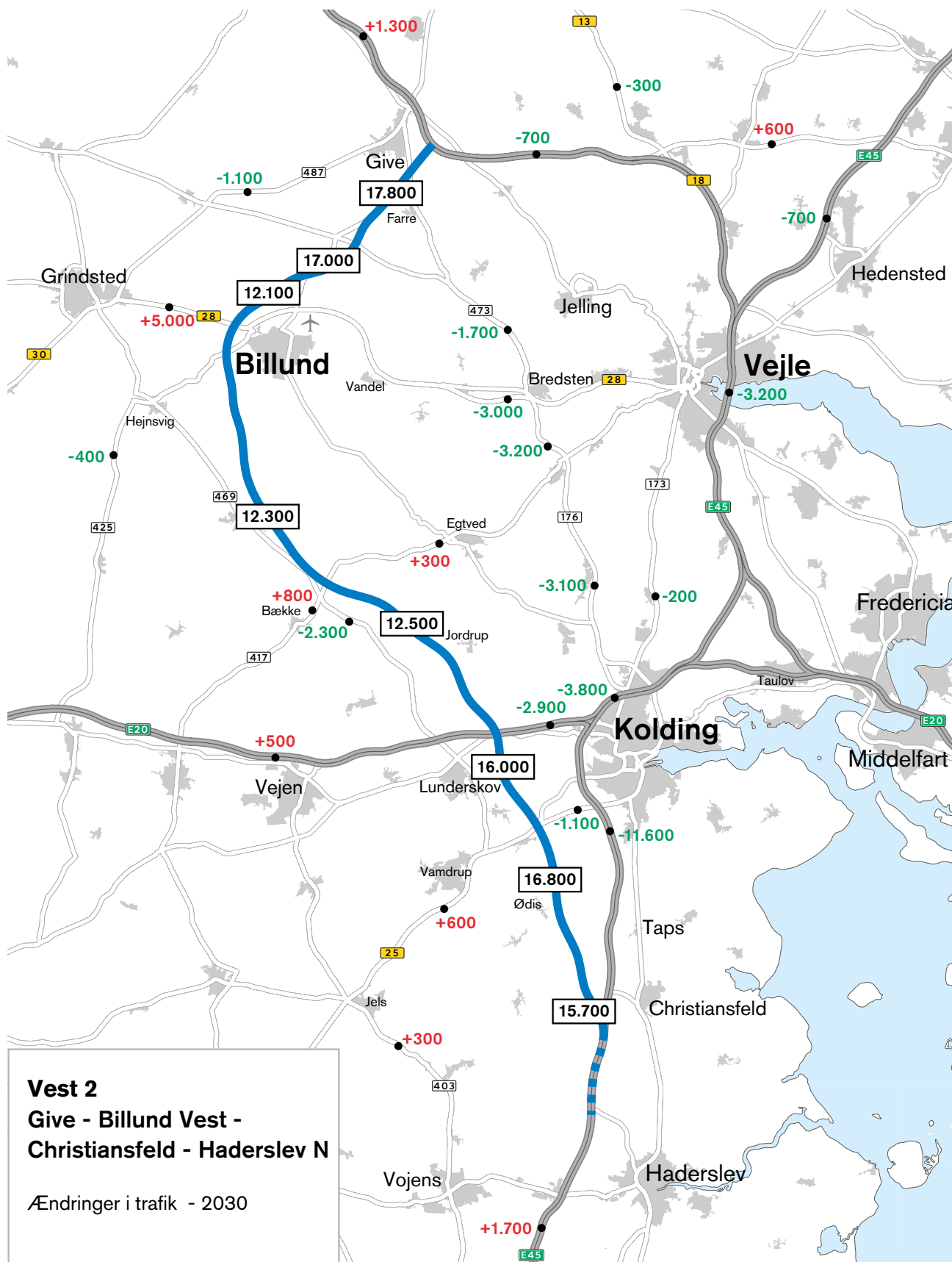
Figur 5.5 Ændring i trafikken i 2030 med forslag Vest 2
