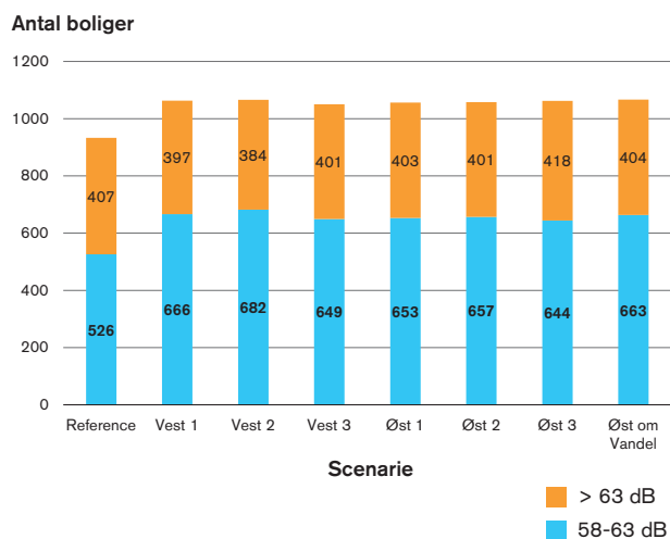
Figur 7.5 Antal boliger i forskellige støjintervaller
