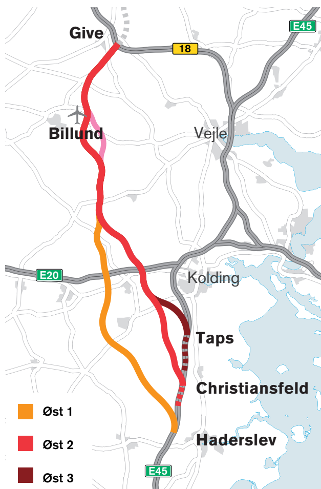
Figur 1.2 Linjeføringer øst om Billund.
