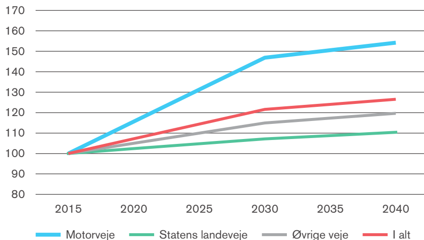
Figur 5.3 Trafikudvikling til 2040 i basisfremskrivning uden Ny Midtjysk Motorvej (indekseret, 2015=100). Udviklingen er baseret på prognoser for 2015, 2030 og 2040. Der er ikke gennemført selvstændige analyser for de mellemliggende år. År 2030 er det åbnings-år der anvendes i analysen og trafikændringer afreporteres som ændring i forhold til basisfremskrivningen. En fremskrivning til 2040 udgør en del af grundlaget for den samfundsøkonomiske analyse, der opgør effekter i årene efter åbning.
