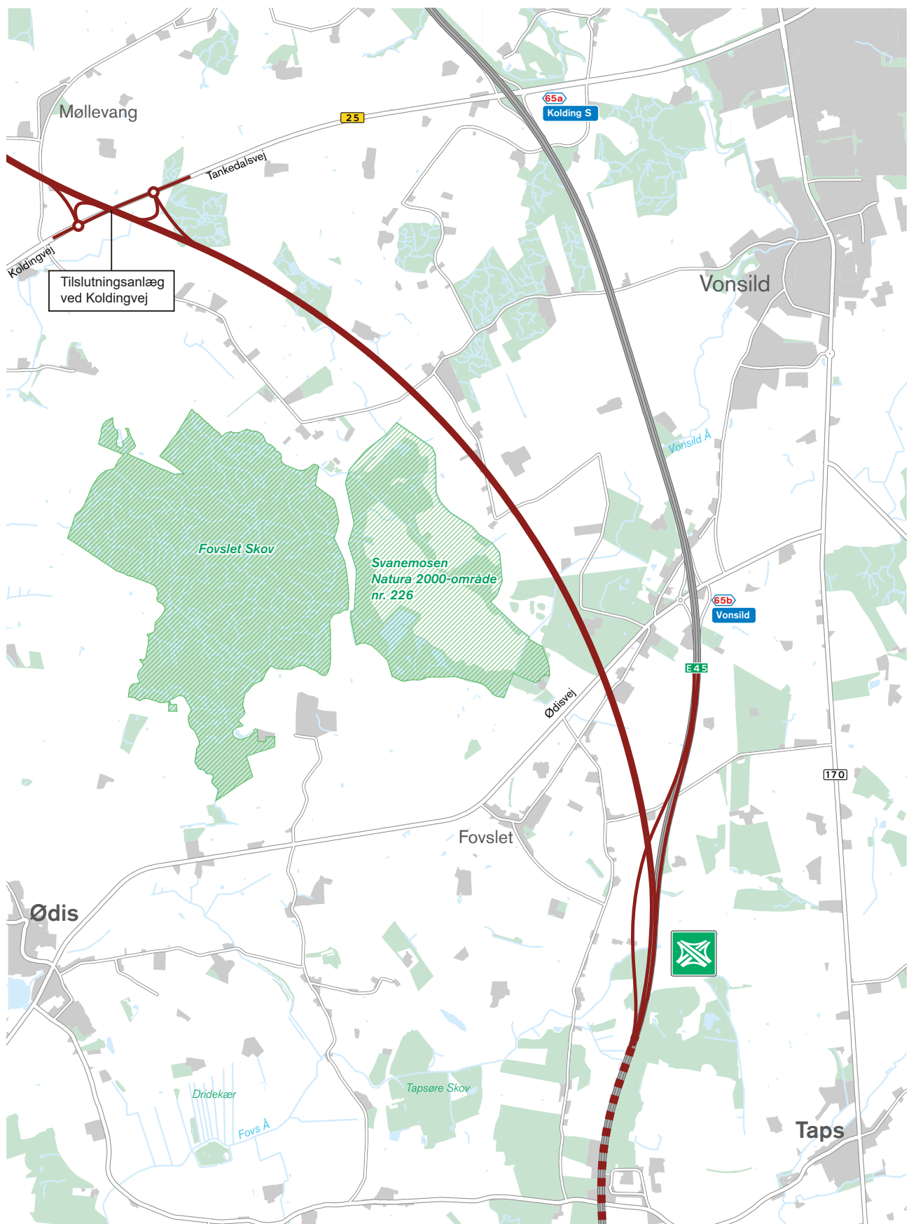
Figur 3.16 Forslag Øst3 mellem Koldingvej og E45
