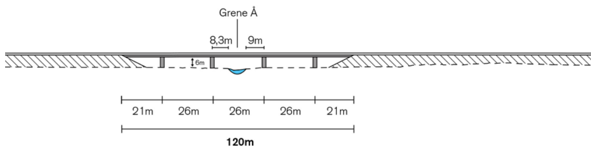
Landskabsbro over Grene Å
