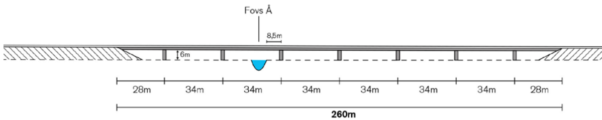
Dalbro over Fovs Å
