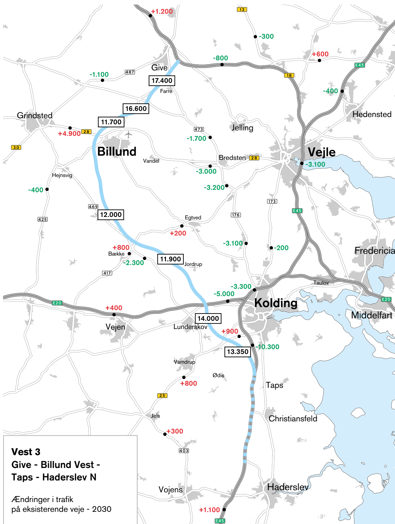
Figur 5.6 Ændring i trafikken i 2030 med forslag Vest 3
