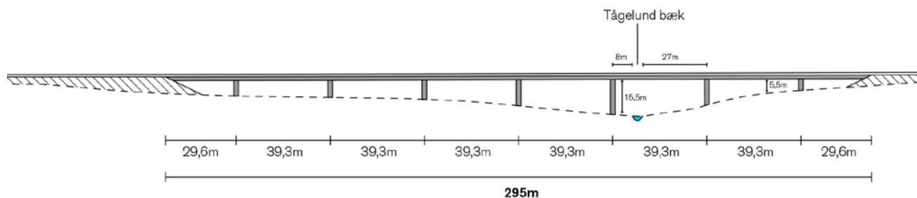
Lang dalbro over Tågelund Bæk
