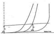
Figur 3 - Lasttankenes grænselinier jf. stk. 6
