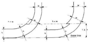
Figur 2 – Brændselsolietankens grænselinjer til brug for stk. 7 og 8
