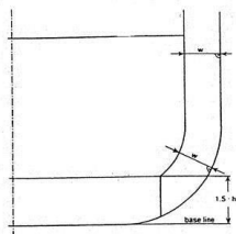
Figur 2 - Lasttankenes grænselinier jf. stk. 4
