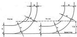
Figur 1 - Lasttankenes grænselinier jf. stk. 3
