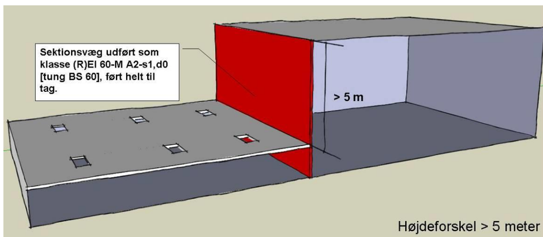
Figur 31: Sikring mod høj-lav brandsmitte, hvor den højere bygnings tag er større end 5 m over den lavere bygnings tag. Ingen krav om brandkam eller brandkamsersætning.
