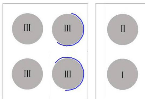
Figur 60: To bassiner med hhv. klasse III tanke og klasse I og II tanke. De to tanke med klasse III væsker, der er i direkte strålingslinie, overrisles hver svarende til \frac{3}{4} tanksvøb (angivet med blåt), i tilfælde af brand i tank med enten klasse I eller klasse II væske. Overrisling af tanke kan undlades, såfremt der i forbindelse med skyggevirksomhed ikke kan forekomme farlig varmepåvirkning på tanken.
