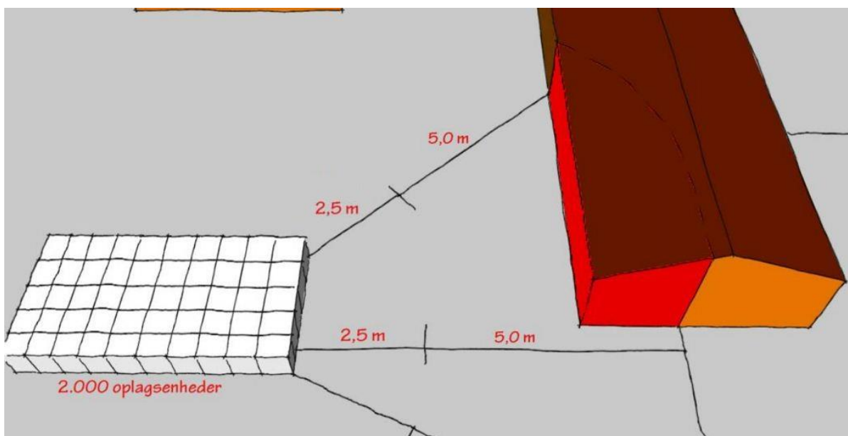
Figur 41: Nedsættelse af den indbyrdes afstand ved oplag mod bygning ved etablering af brandsektionsadskillelse i facaden inden for den krævede afstand (i dette eksempel 7,5 m). Sikring af tag og særlige foranstaltninger mod brandsmitte på gavlvæggen skal kun ske, når den indbyrdes afstand er mindre end 5 m.
