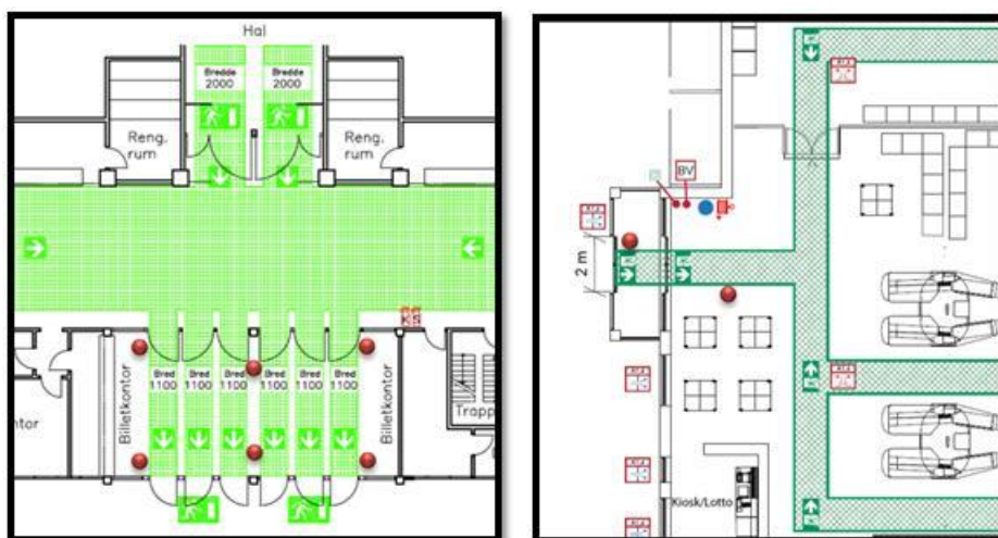
Figur 61: To eksempler på placering af håndspritdispensere uden for flugtveje. De grønne områder illustrerer friarealer/flugtvejspassager. Placeringerne af håndspritdispensere er markeret med røde prikker. Eksemplet til venstre viser indgangsområdet til en stor hal/arena. Eksemplet til højre viser indgangsområdet til en større butik.
