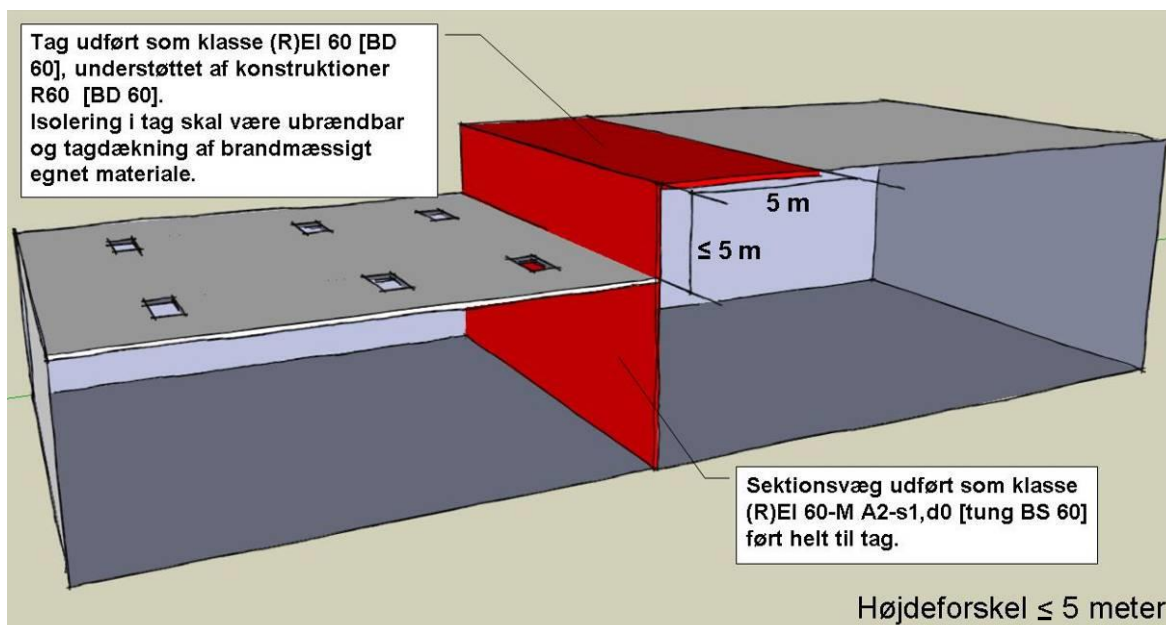
Figur 30: Sikring mod høj-lav brandsmitte, hvor den højere bygnings tag er mindre end eller lig med 5 m over den lavere bygnings tag. Løsning med brandkamsersætning. Der henvises til vejledningens afsnit om brandkamsersætning for udførelse af tagdækning i brandmæssigt egnet materiale.
