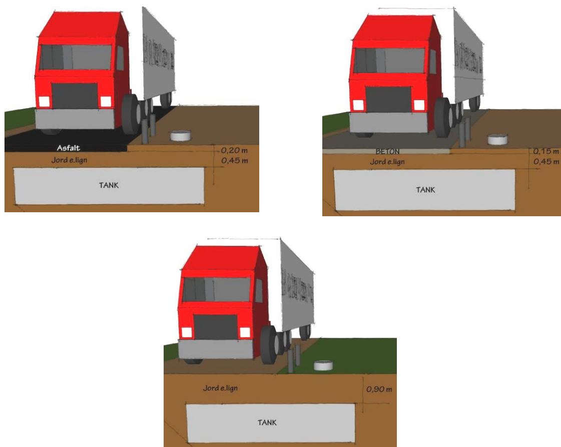
Figur 14: Illustration af forskellige belægninger, herunder tykkelse til beskyttelse af tanken mod trafiklast.
