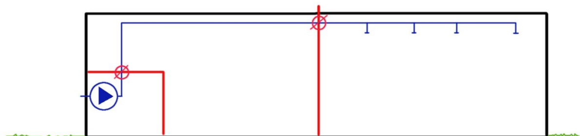
Figur 18: Eksempel på et ventilationsanlæg, der betjener én brandsektion med oplag af kategori A-væsker (må kun betjene én brandsektion). Kanal gennemføringen mellem brandsektionerne og mellem ventilationsrummet og brandsektion er sikret med et brand- og røgspjæld (BRS-spjæld). Kanalerne er udført af mindst materiale klasse A2-s1,d0 af metal med et smeltepunkt på mindst 850 °C.
