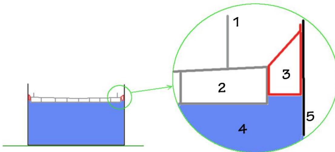
Figur 58: Skitseret detalje af flydetagets forbindelse til tankens inderside: 1. Skumbarriere, 2. Hulrum i Double Deck, 3. Rim-seal, 4. Væske, 5. Tanksiden.
