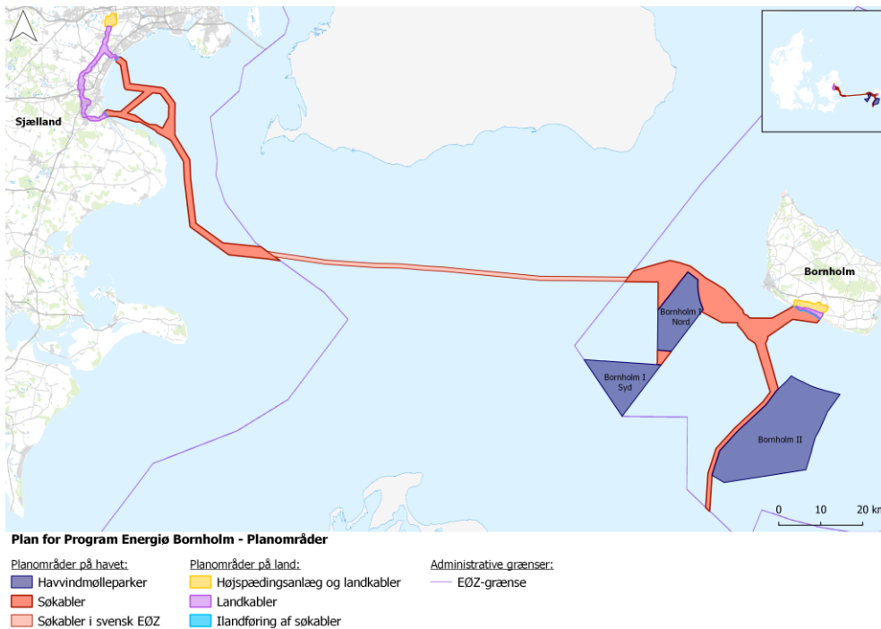
Figur 1 Oversigt over områder i Udkast til Plan for Program Energiø Bornholm. Områder på havet til kabelkorridor gennem svensk farvand (EØZ) er ikke omfattet af planen.
