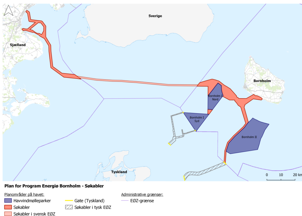
Figur 4 Områder til søkabler i Plan for Program Energiø Bornholm, samt områder til søkabler gennem svensk farvand og potentielle områder til søkabler i tysk farvand. Søkabler i udlandet er ikke omfattet af planen.
