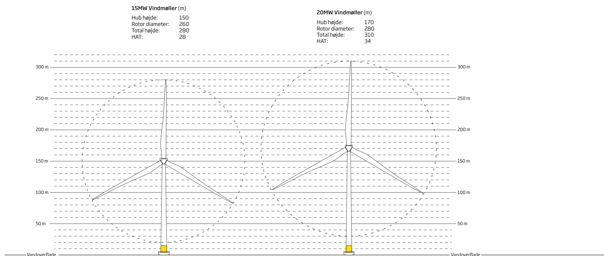
Figur 3: Vindmølledimensioner
