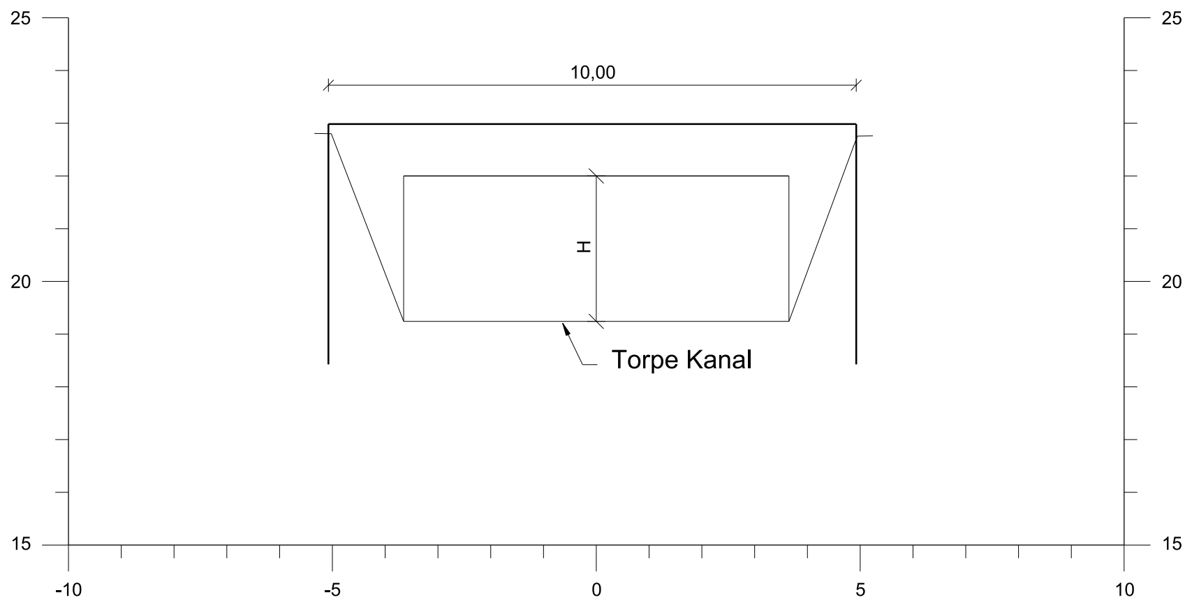
SECTION A-A 1:100 St. 78+484.557
