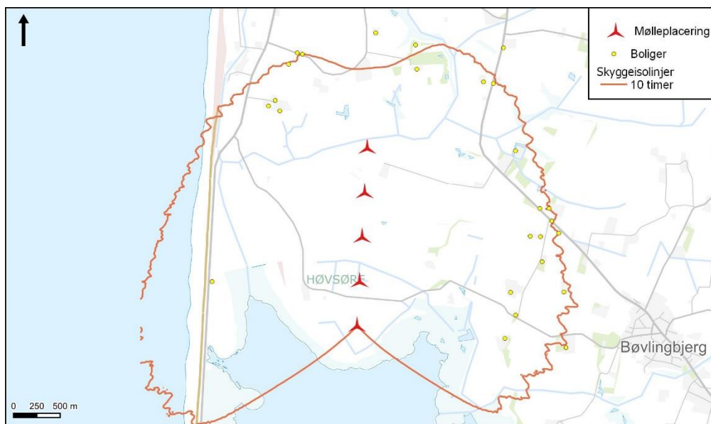
Figur 9.3: Beregning af antal timer pr. år med reelt skyggekast omkring de nye prototypevindmøller ved Høvsøre.
