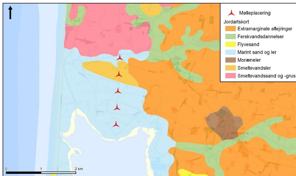
Figur 15.2 Jordartskort 1:200.000 (DGU, 1989).
