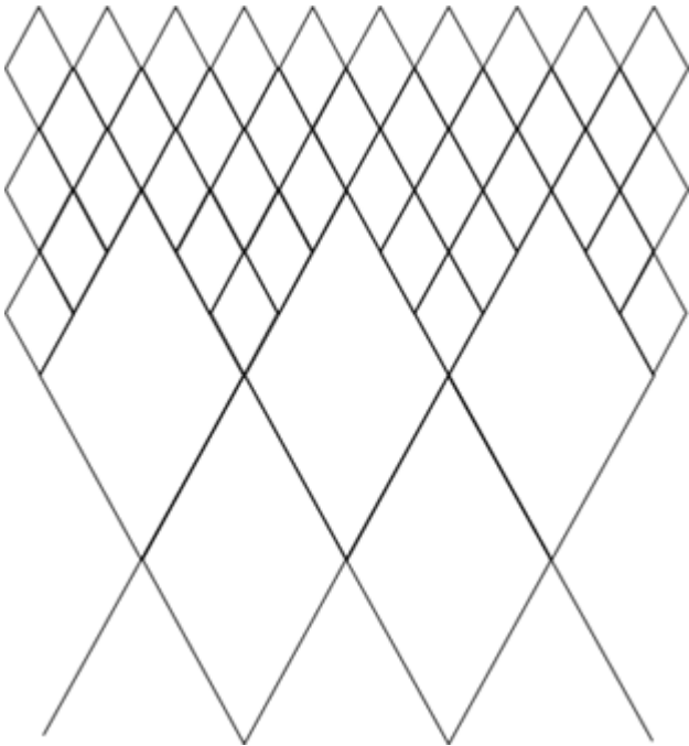
Figur 4. Illustration af sammenføjning af tre 90-100 mm. masker med én 270 mm. maske
