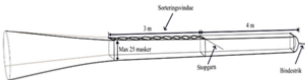
Figur 3. fire-panel fangstpose med et selektionspanel med diamantmasker på mindst 270 mm
