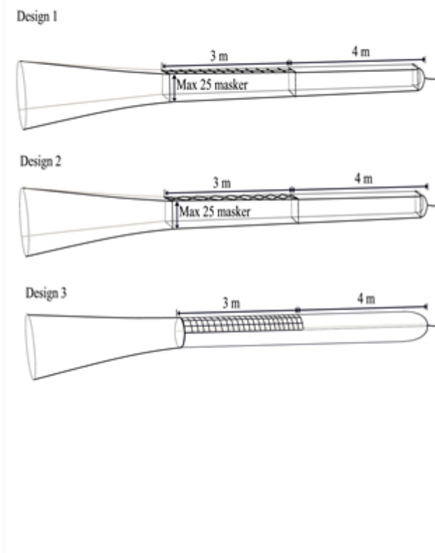
Figur 4. Illustration af sammenføjning af tre 90-100 mm. masker med én 270 mm. maske
