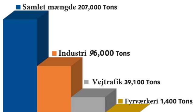
MÆNGDE FINSTØV I TYSKLAND/ÅR (STATUS 2018)
