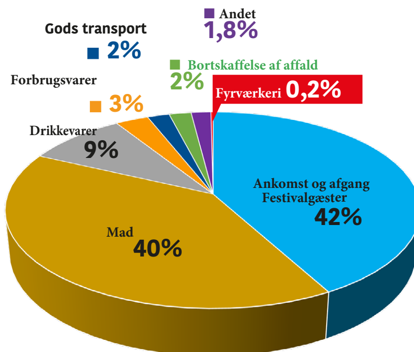
CO2E-EMISSIONER FRA ZÜRI FÄSCHTS (MYCLIMAT)
