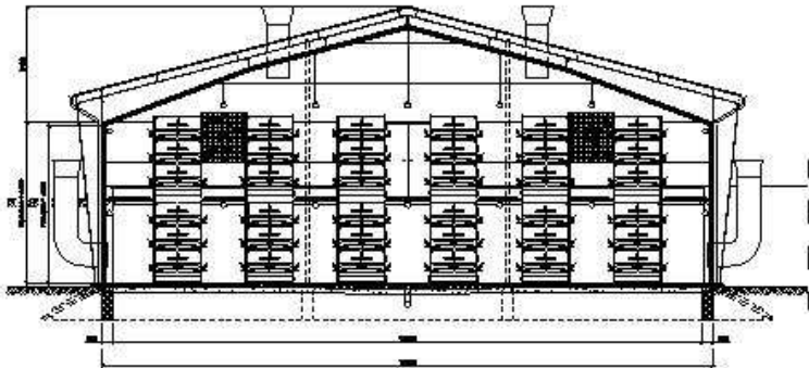
Tværsnit af bursystem med 2 x 3 etager
