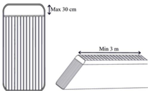
Figur 1. Rejerist med tunnel, jf. nr. 1.
