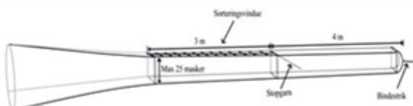
Figur 1. 4-panel fangstpose med et 180 mm kvadratmasket selektionspanel
