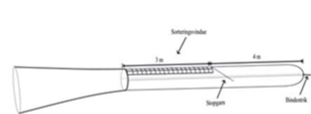
Figur 5. 2-panel fangstpose med et 180 mm kvadratmasket selektionspanel
